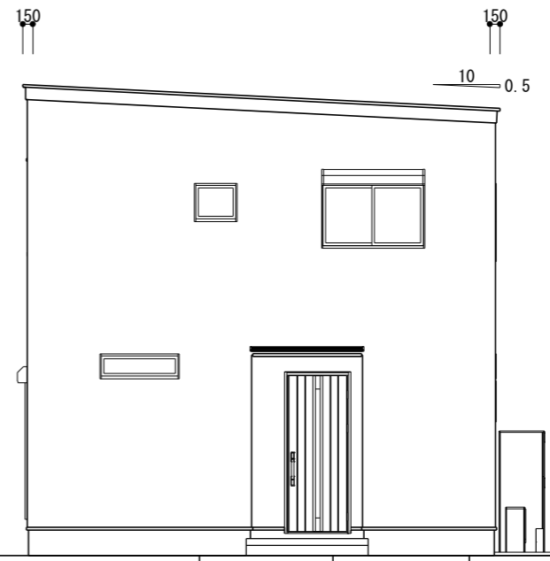
東立面図 S=1/100
