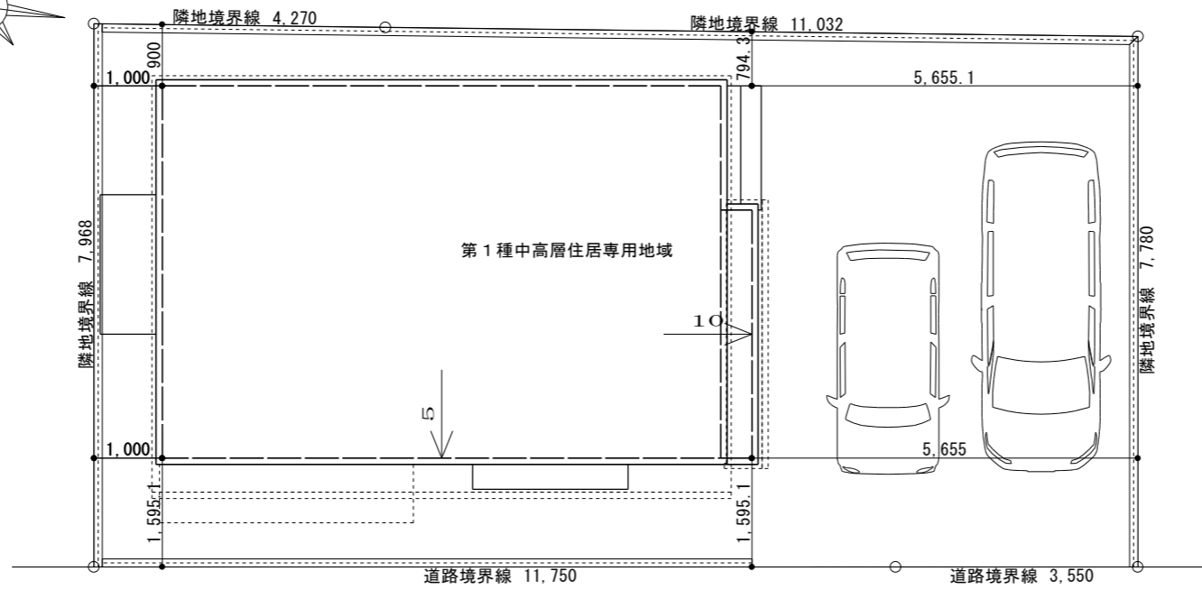
配置図 S=1/100
