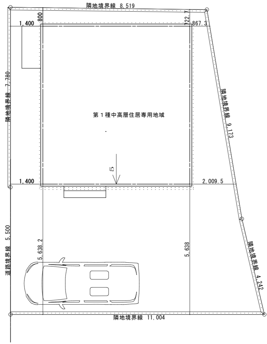
配置図 S=1/100
