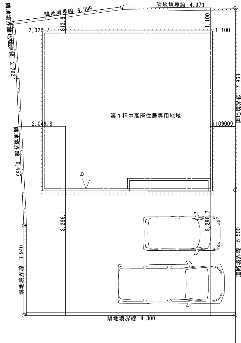
配置図 S=1/100
