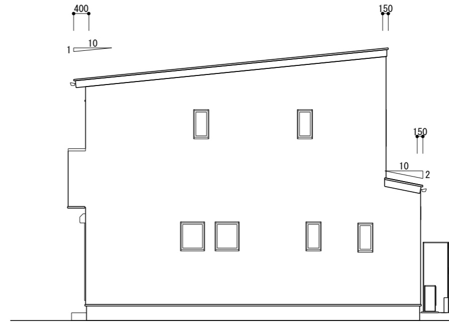
東立面图 S=1/100
