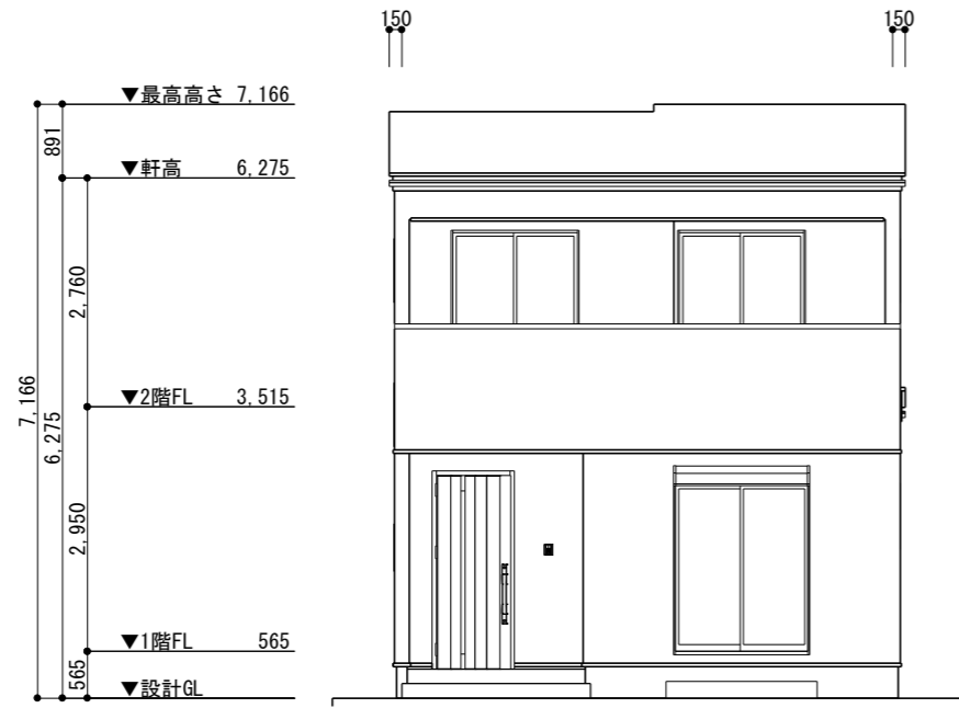
南立面图 S=1/100
