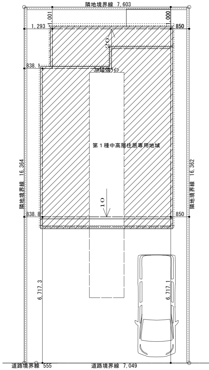
配置図 S=1/100
