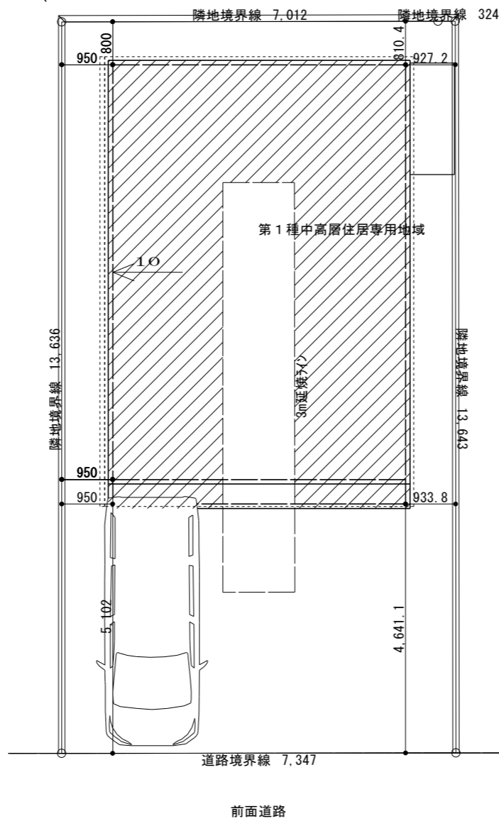
配置図 S=1/100
