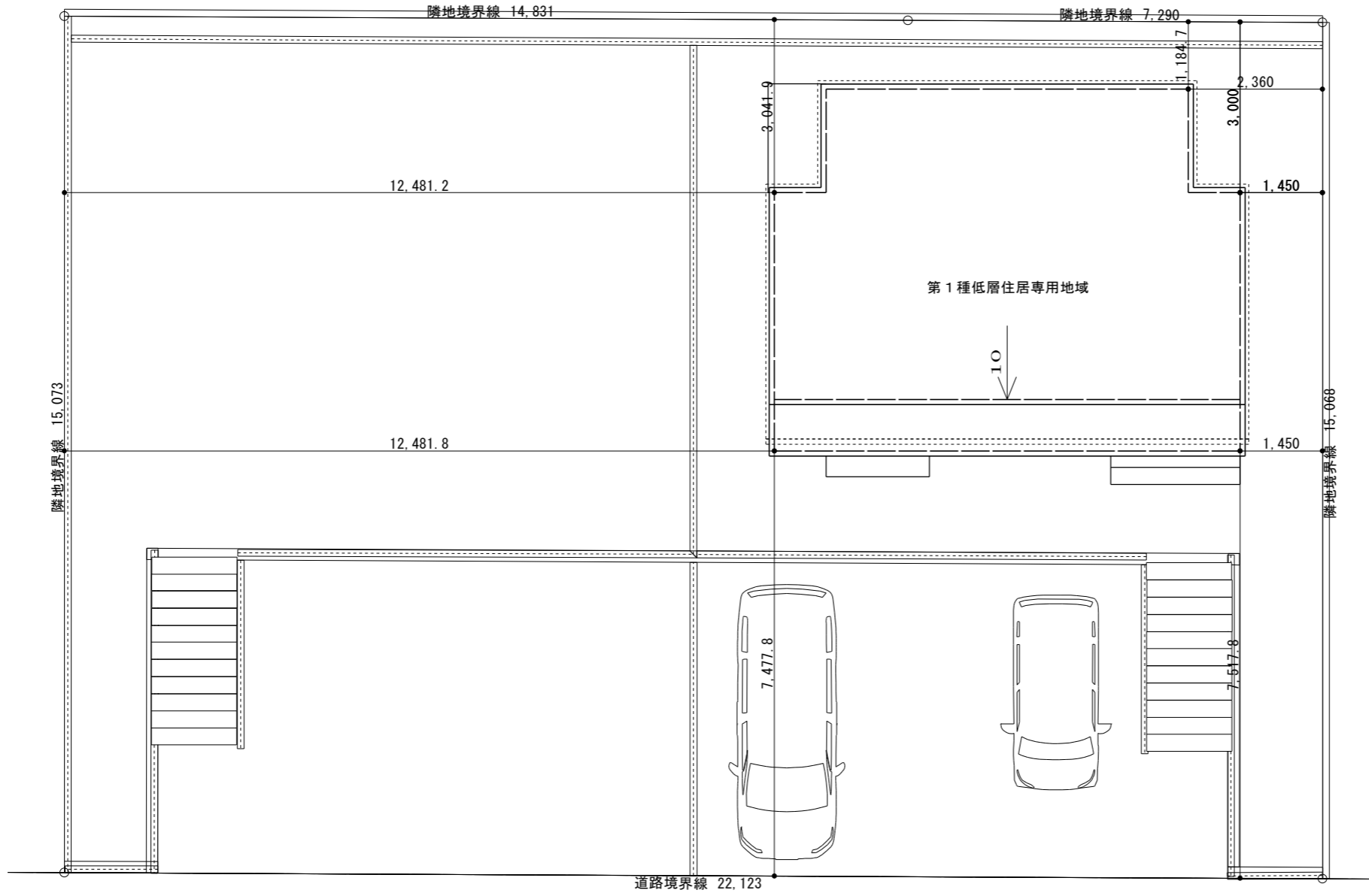
配置図 S=1/100
