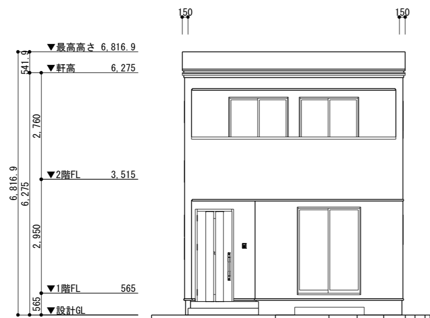
南立面図 S=1/100
