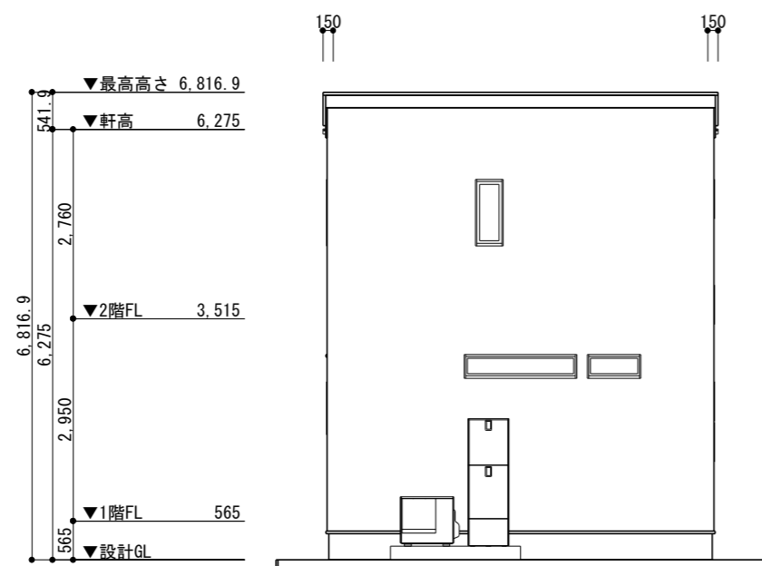
北立面図 S=1/100
