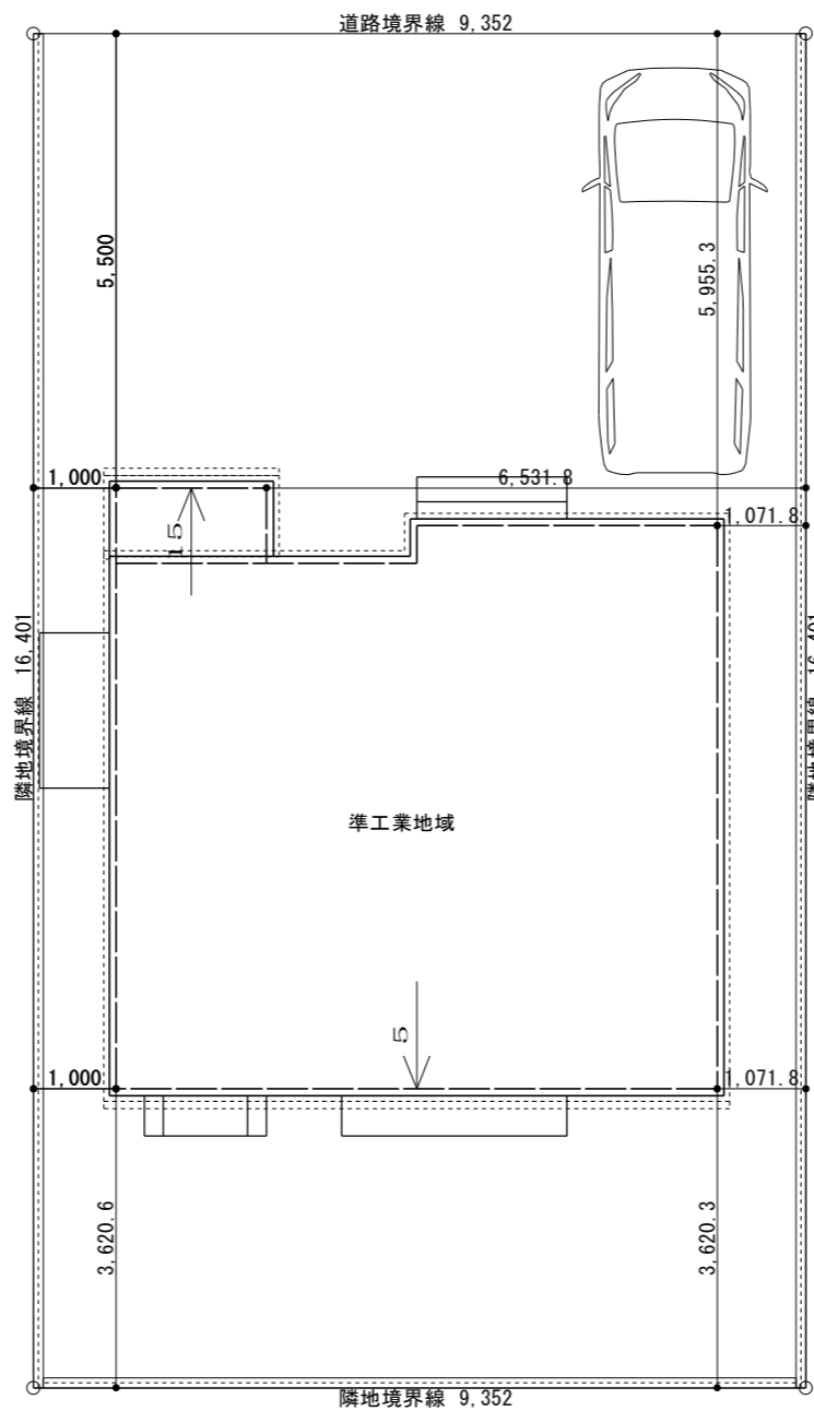
配置図 S=1/100
