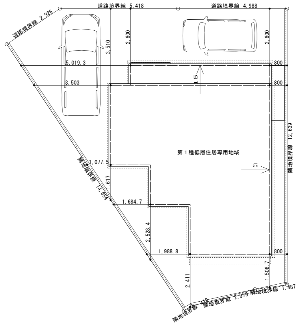
配置図 S=1/100
