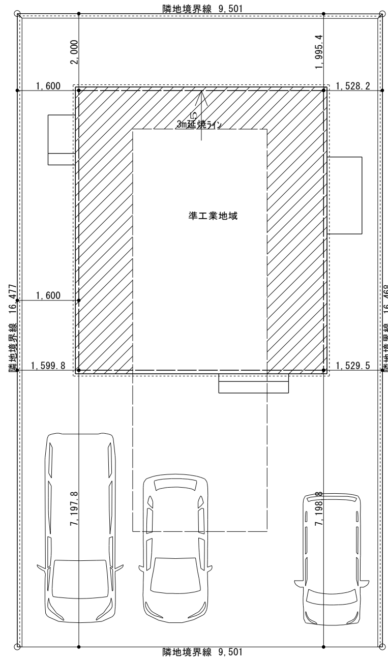
配置図 S=1/100
