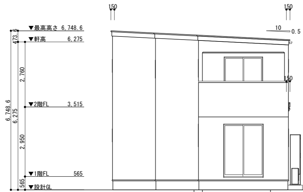
南立面图 S=1/100
