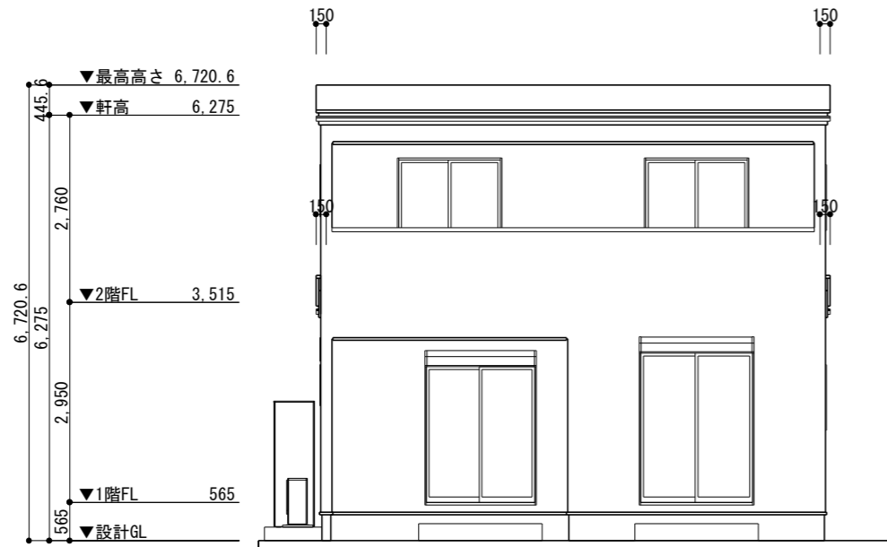
南立面图 S=1/100
