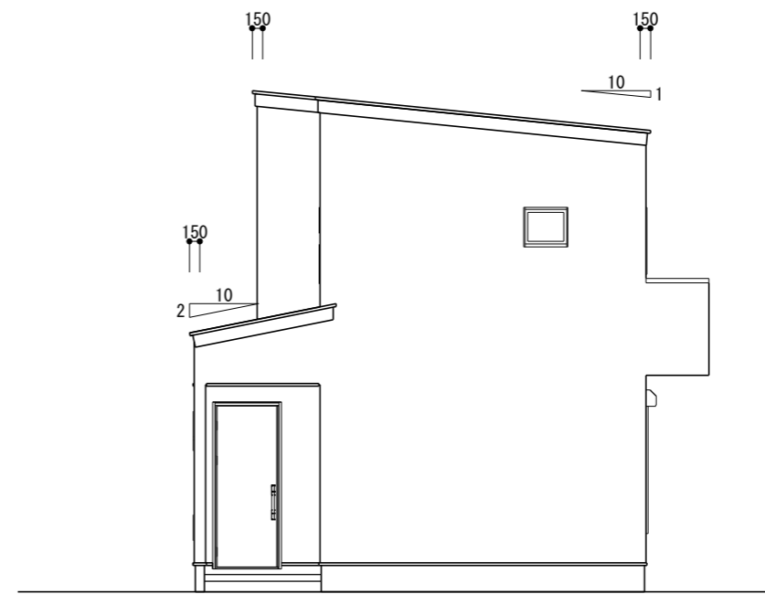
西立面図 S=1/100
