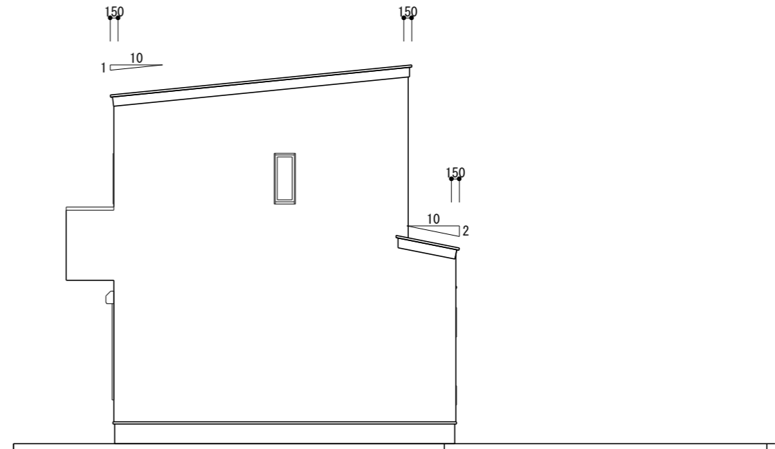
東立面図 S=1/100
