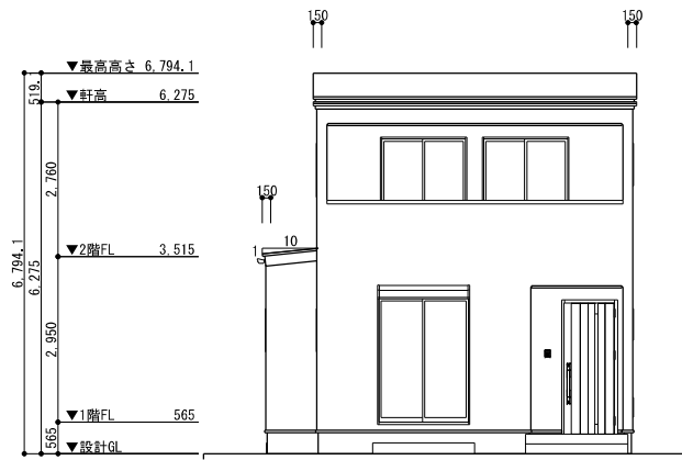
南立面図 S=1/100
