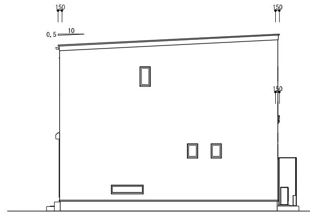
東立面図 S=1/100
