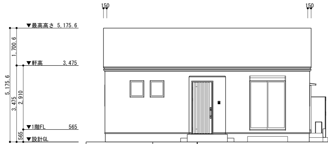
南立面图 S=1/100
