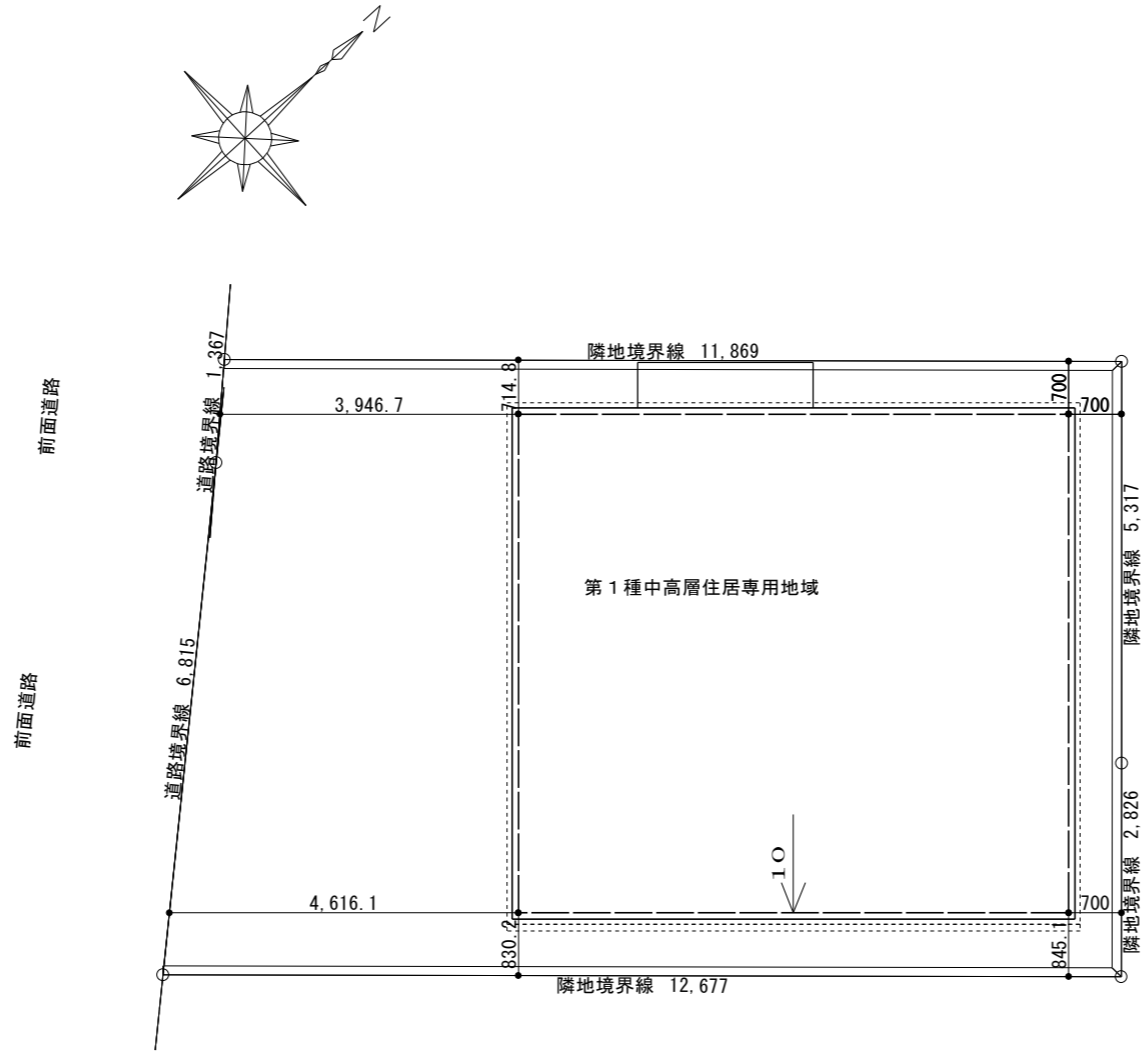
配置図 S=1/100
