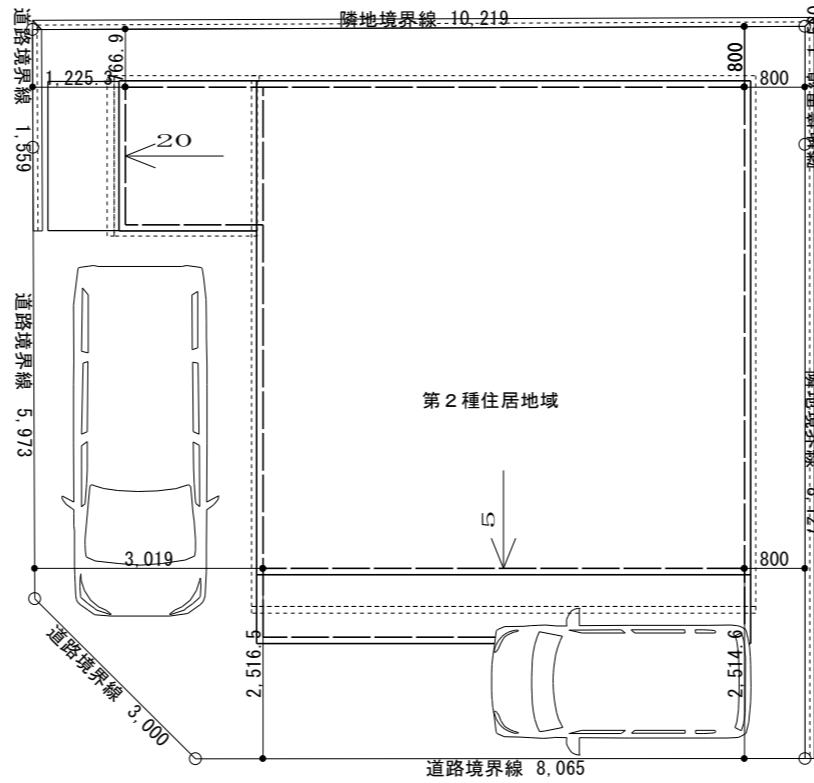
配置図 S=1/100
