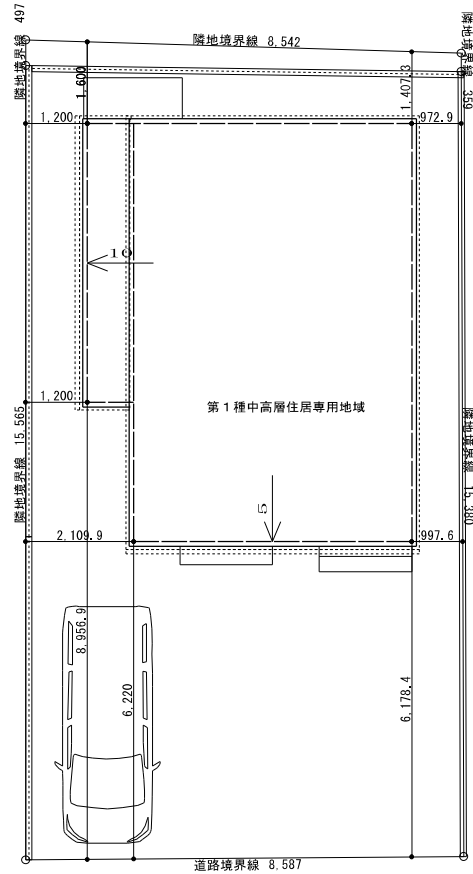
配置図 S=1/100
