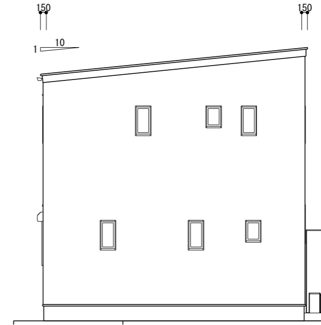
東立面図 S=1/100
