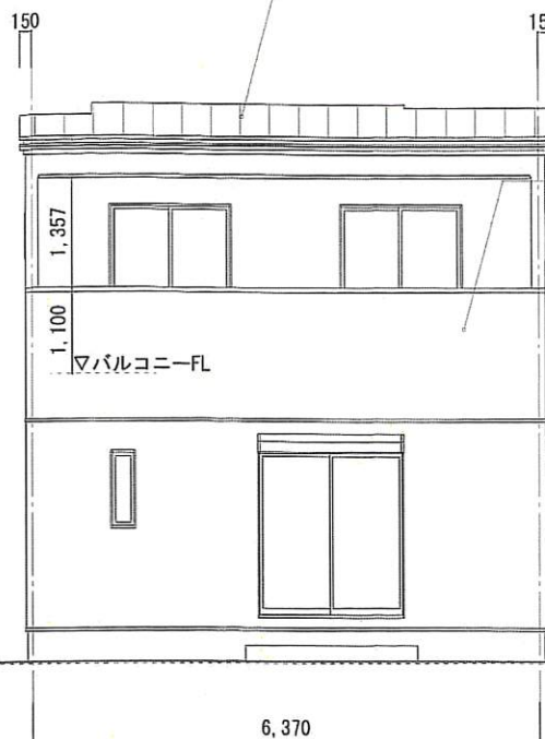
南立面図 S=1/100
