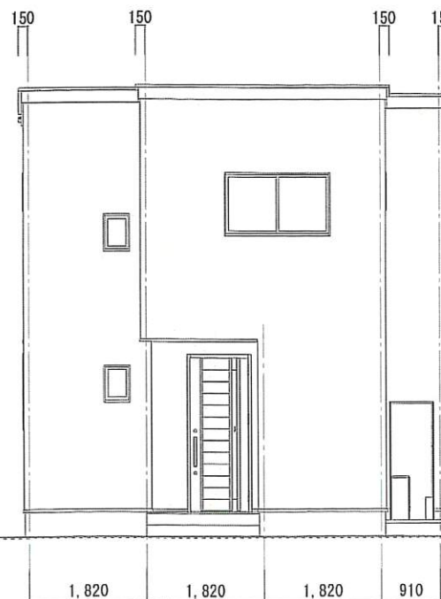
北立面図 S=1/100
